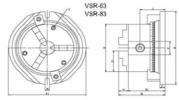
VSR-63 + VSC-6A 3JAW CHUCK VSR-83 + VSC-8A 3JAW CHUCK
